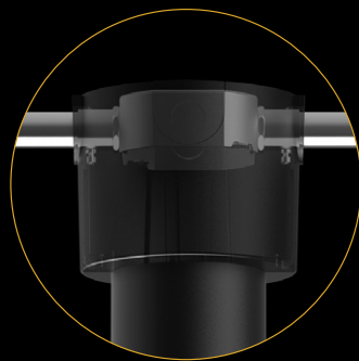
CONDUIT CANOPY (Conceals J-Box / conduit connections)
