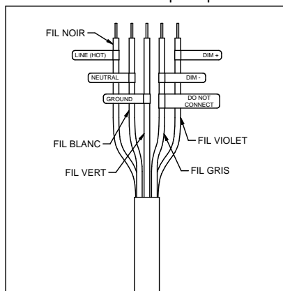
STANDARD OU DM1
