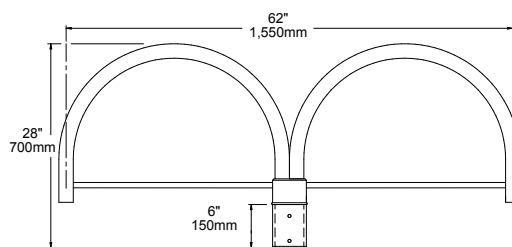
SLA18-2 (4" pole)
