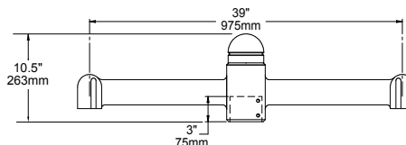
SLA20-2 (4" pole)
