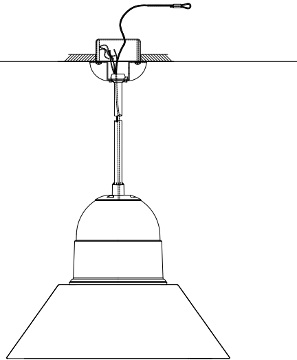
* Pendant Mount
